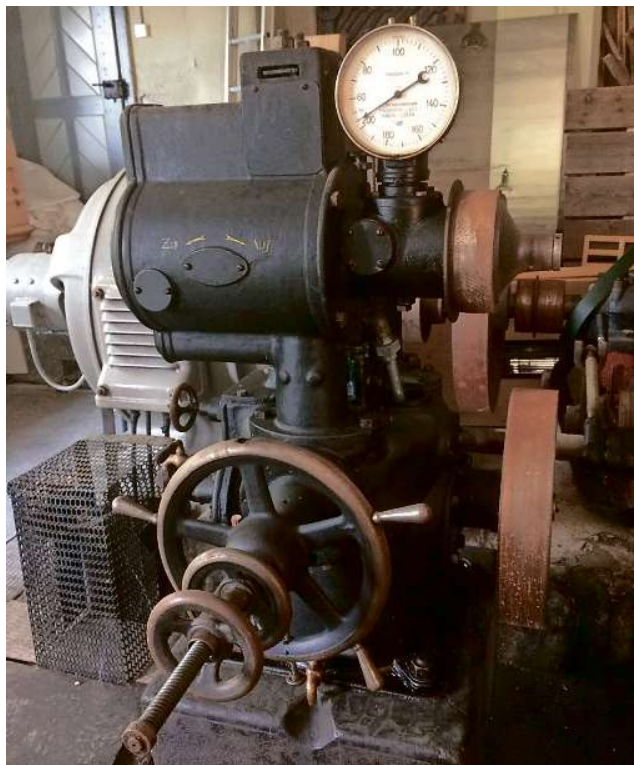
Die Turbine aus dem Jahr 1905 soll restauriert werden.
